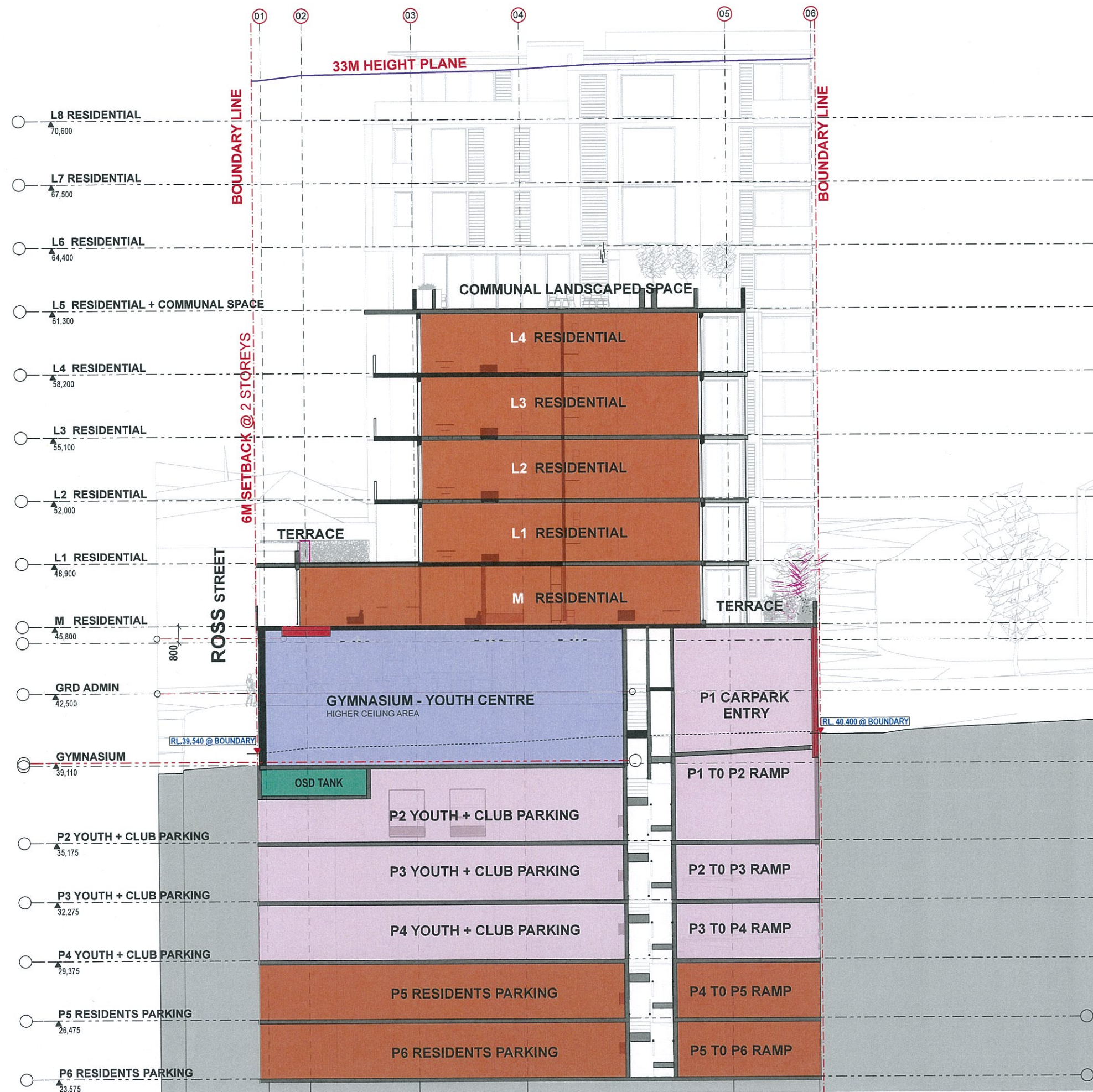
CROSS SECTION (A-A)
